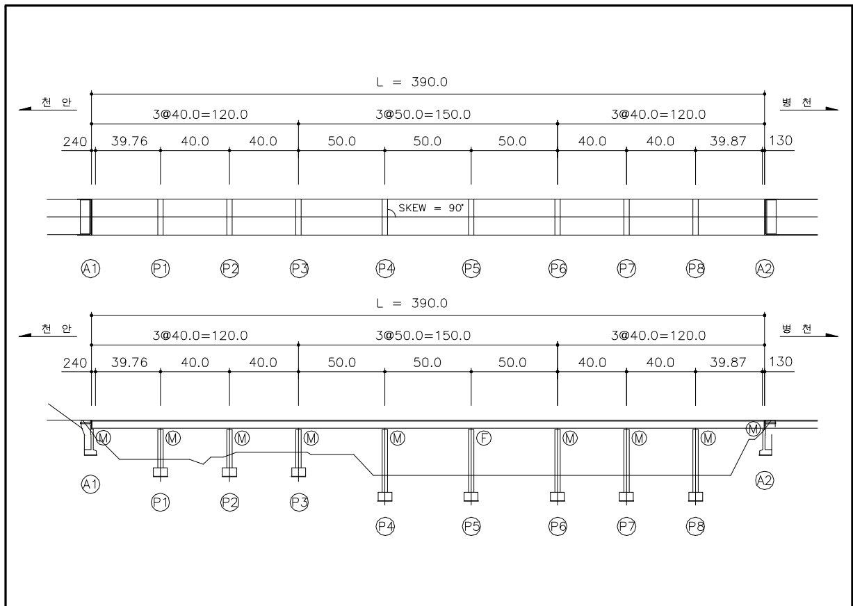
<그림 6.1> 목주교 종평면도
